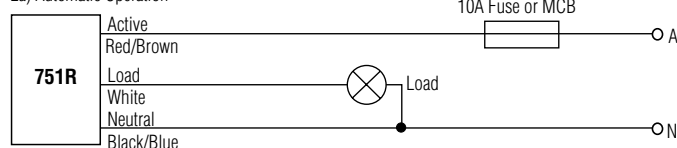
2a) Automatic Operation
