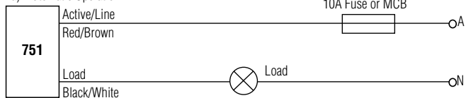
1a) Automatic Operation
